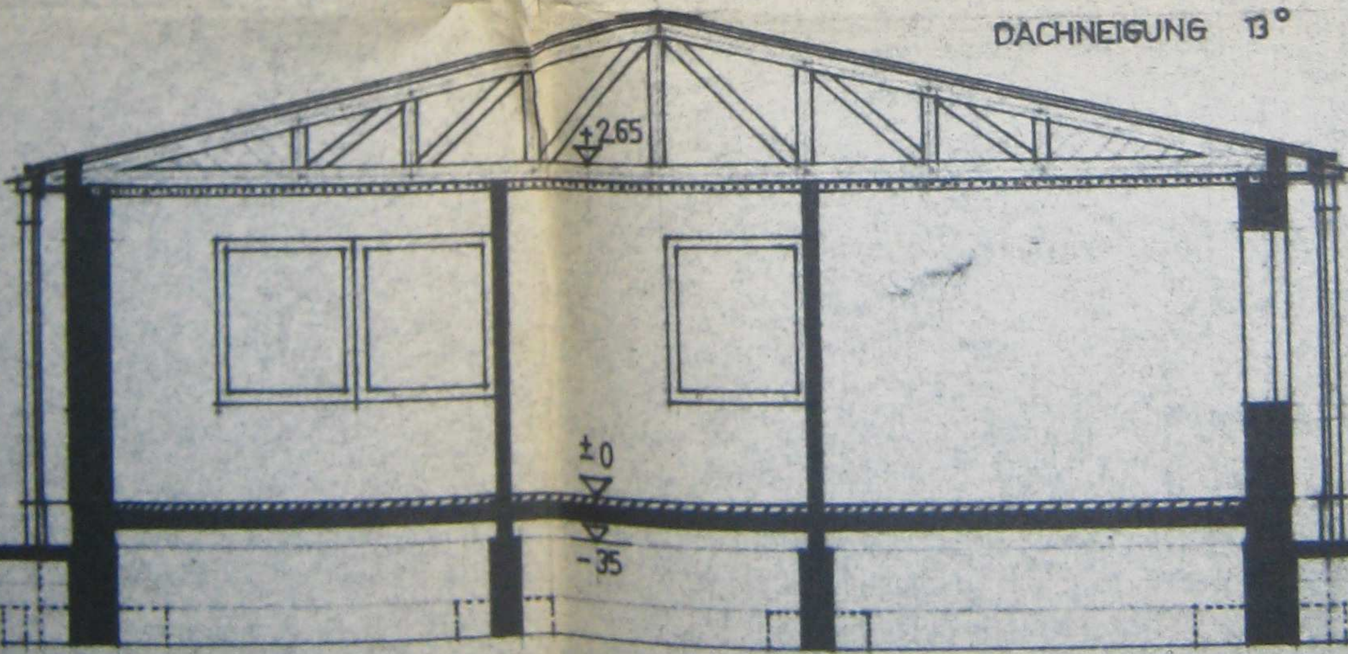
SCHNITT 1 — 1
